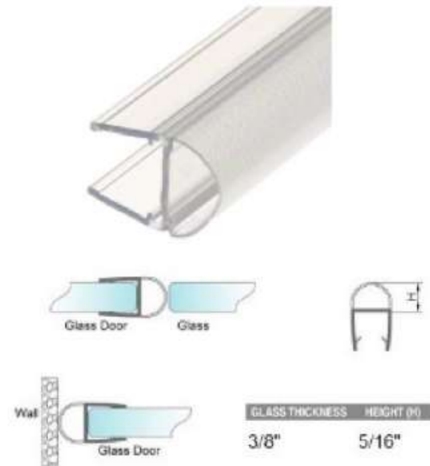
PVC-24
